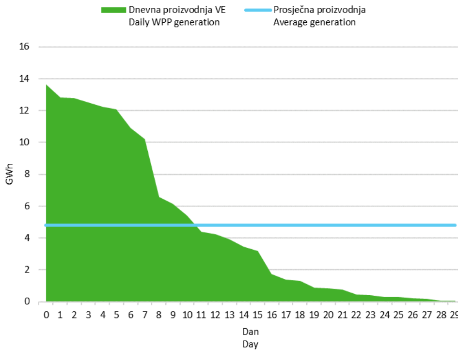
Slika 6 Krivulja trajanja dnevne proizvodnje vjetroelektrana u studenom 2020. godine
