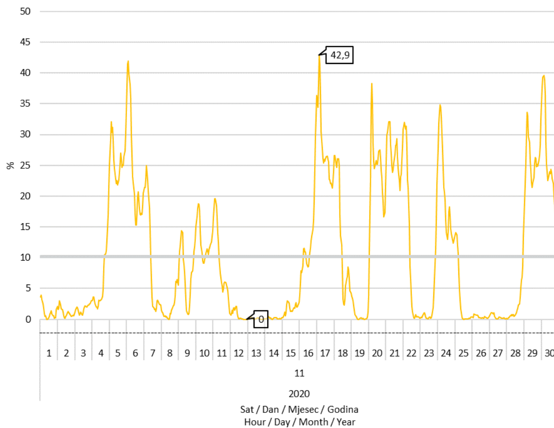
Slika 8 Udio proizvodnje vjetroelektrana u pokrivanju satnog opterećenja elektroenergetskog sustava u studenom 2020. godine
