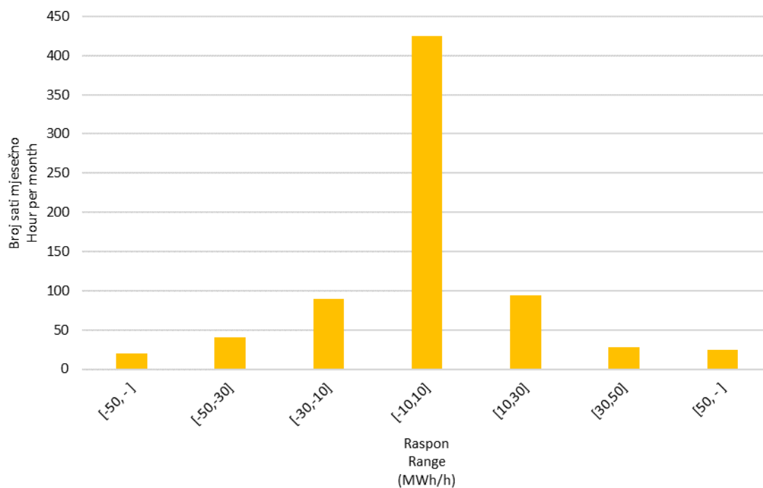
Slika 10 Statistička raspodjela satnih promjena proizvodnje VE u studenom 2020. godine
