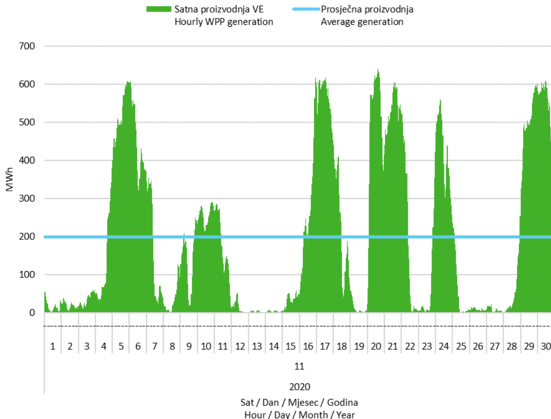
Slika 2 Satna proizvodnja svih vjetroelektrana u studenom 2020. godine
