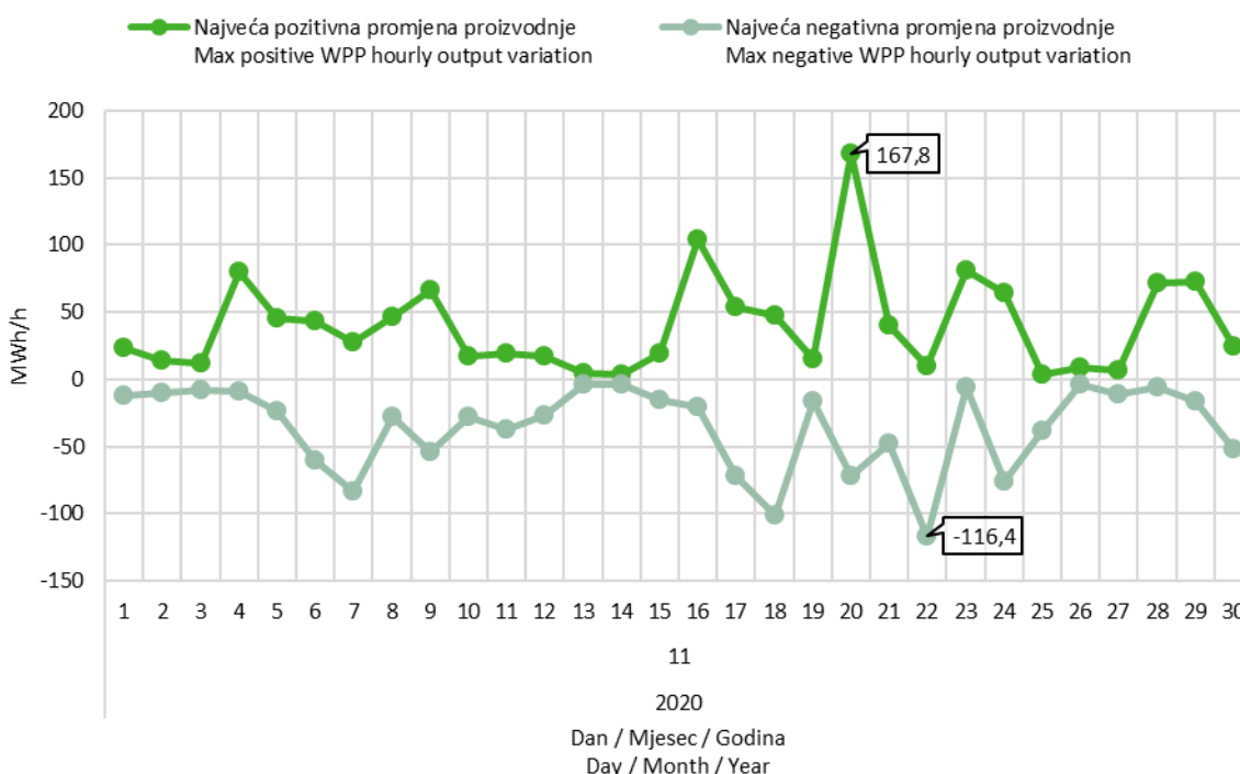
Slika 9 Maksimalna pozitivna i maksimalna negativna promjena satne proizvodnje VE u studenom 2020. godine
