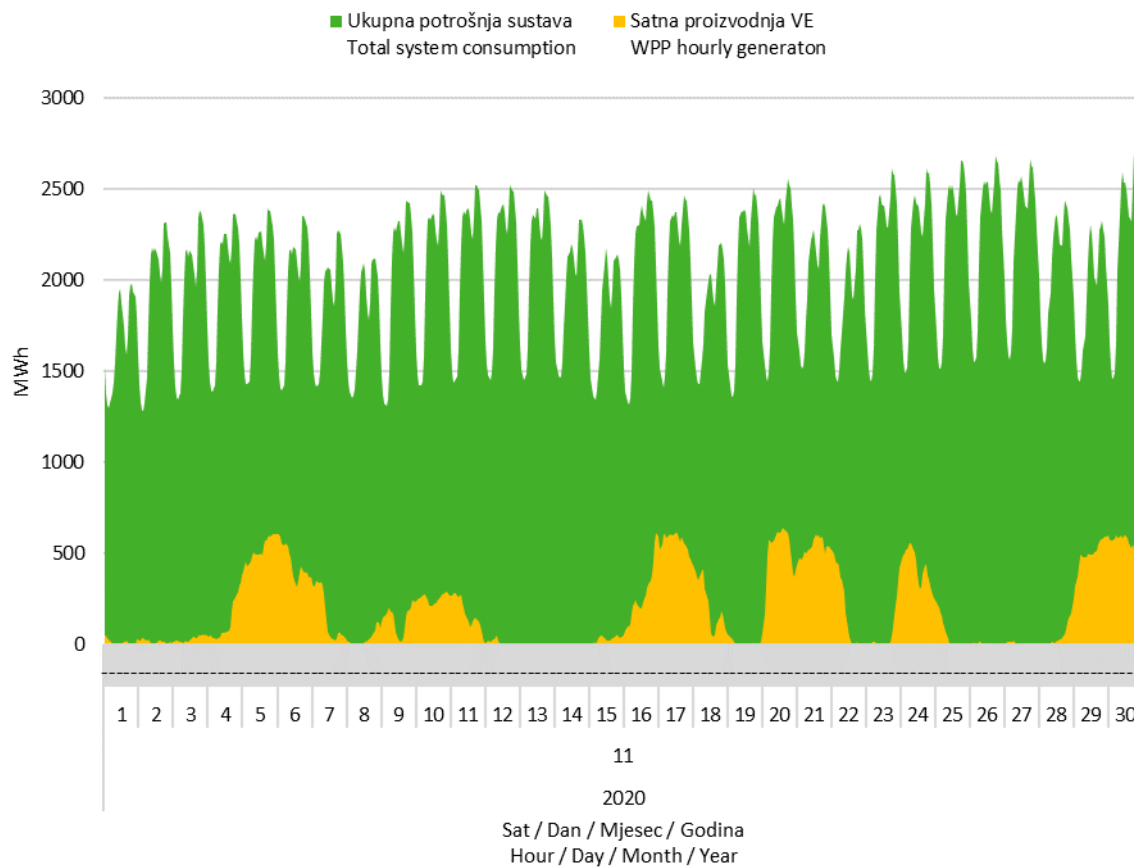
Slika 7 Usporedba satnog dijagrama opterećenja sustava i proizvodnje vjetroelektrana u studenom 2020. godine
