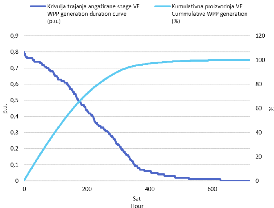
Slika 3 Krivulja trajanja angažirane snage svih VE i kumulativna proizvodnja VE u studenom 2020. godine u jediničnim vrijednostima
